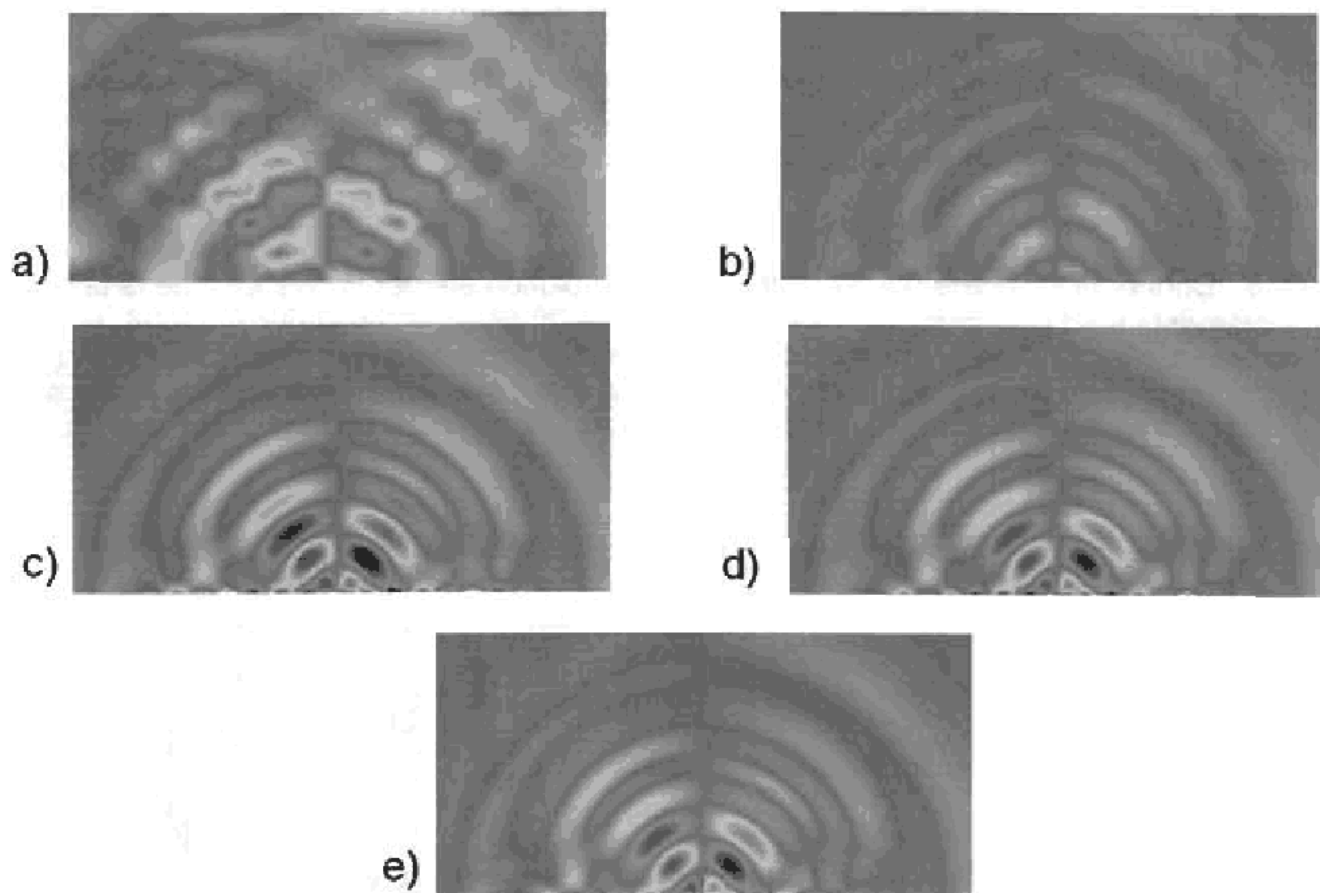
Figure 23 : déplacement selon \vec{x} pour différentes tailles d'éléments.
