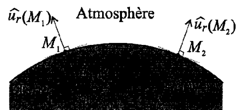
FIGURE 1 — Structure géométrique du champ électrique terrestre
