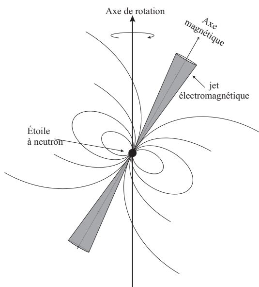
FIG. 1 – Schéma d'un pulsar.
