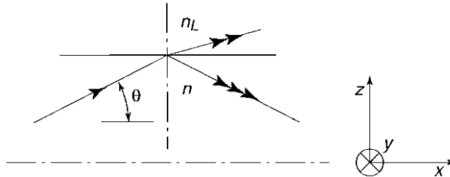
FIG. 2: Autofocalisation du faisceau – Rayon(s) réfléchi et/ou réfracté.
